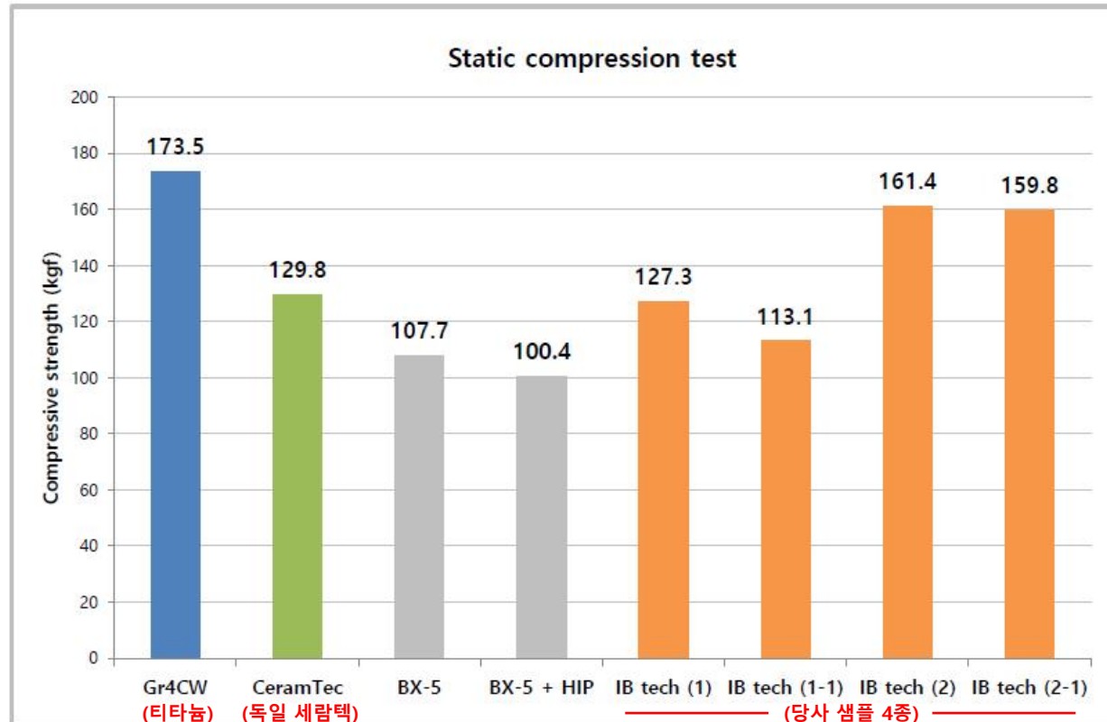
압축강도 테스트
